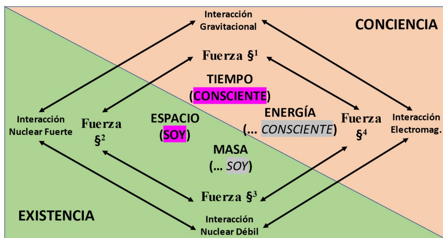
Figure 3. Correspondencia estructural entre los componentes y fuerzas de las cuerdas de conciencia / existencia y las partículas e interacciones fundamentales de la física.
